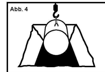
* Tankhöhe + 15 cm Sandbett
