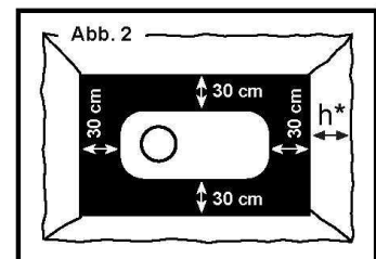
Bei der Verwendung einer Domverlängerung und / oder eines Schiebedoms muß die Tiefe der Grube entsprechend verändert werden.
